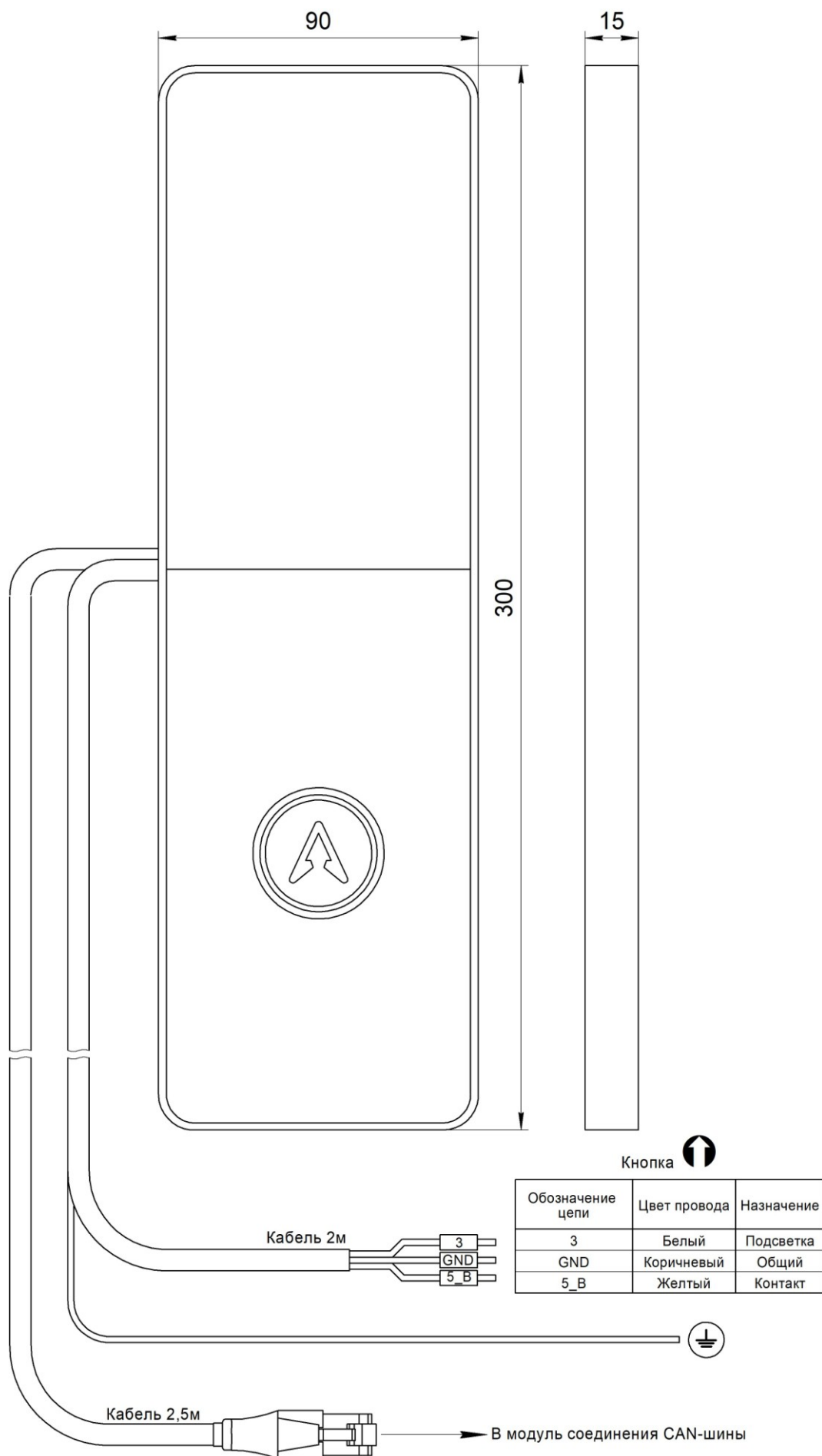
Рис.1 Внешний вид Вызывной пост ОПАЛ (жгут RJ45) НШЕК.468381.056
